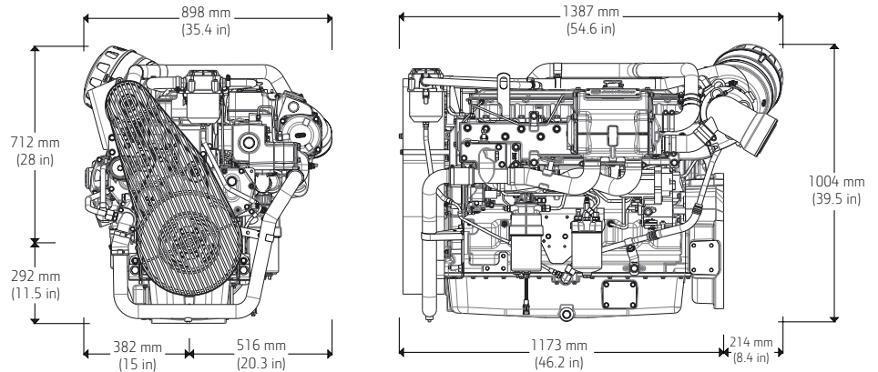
6068AFM shown
